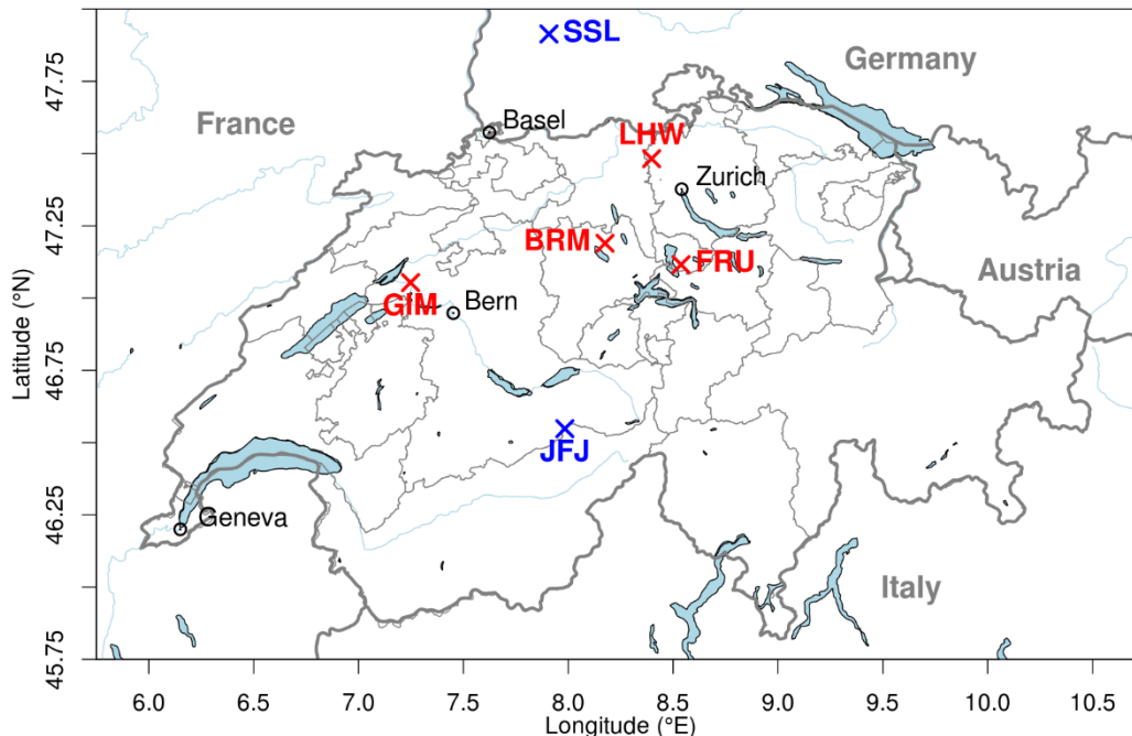
Abbildung 37: Übersicht über das Messnetz von CarboCount CH (rot) mit den vier Standorten Lägern-Hochwacht (LHW, seit Aug. 2012), Beromünster (BRM, seit Nov. 2012), Frübüel (FRU, Nov. 2012-Dez. 2015) und Gimmiz (GIM, seit Feb. 2013) sowie weiteren Messstellen (blau; Jungfrauoch, JFJ; Schauinsland, SSL).
