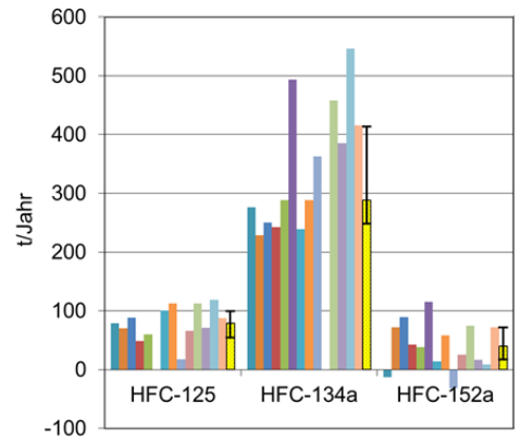
Abbildung A2: Grafische Darstellung der Auswahlkriterien und des Vorgehens zur Bestimmung der Emissionen halogenierter Spurengase der Schweiz (im Jahr 2020 mit 12 Fällen).
