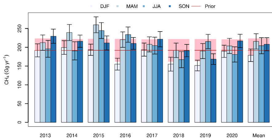
Abbildung 41: Totale saisonale Methanemissionen in der Schweiz (DJF: Dezember, Januar, Februar; MAM: März, April, Mai; JJA: Juni, Juli, August; SON: September, Oktober, November). A priori Werte und deren Unsicherheiten sind als rote Linie und schattierte Fläche gezeigt, während die Resultate der inversen Modellierung als blaue Balken gezeigt sind.
