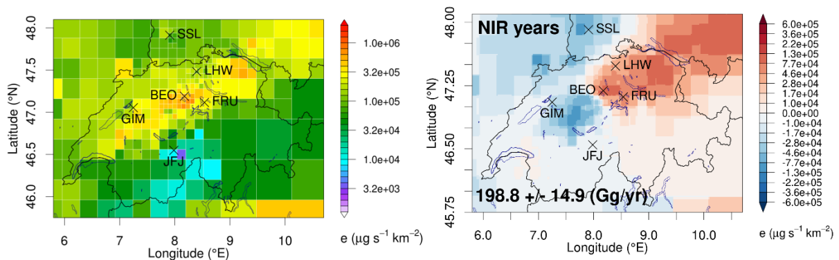
Abbildung 38: Links; räumliche Verteilung der Schweizer \text{CH}_4 Emissionen nach Hiller et al. (2014); Rechts; Emissionsdifferenz der aus der inversen Modellierung gewonnenen Verteilung als Mittel für die Jahre 2013-2019. Dabei weisen blaue (rote) Regionen auf geringere (stärkere) Emissionen als im Inventar hin.
