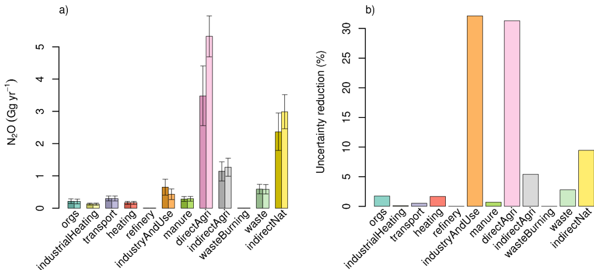
Abbildung 45: (links) mittlere Schweizer N 2 O Emissionen nach Emissionssektor für die Jahre 2017-2020 und über alle Sensitivitätsinversionen. A priori Werte sind als dunklere Färbung angegeben. Fehlerbalken repräsentieren 1- \sigma Konfidenzbereiche. (rechts) Unsicherheitsreduktion zwischen a priori und a posteriori Emissionen.
