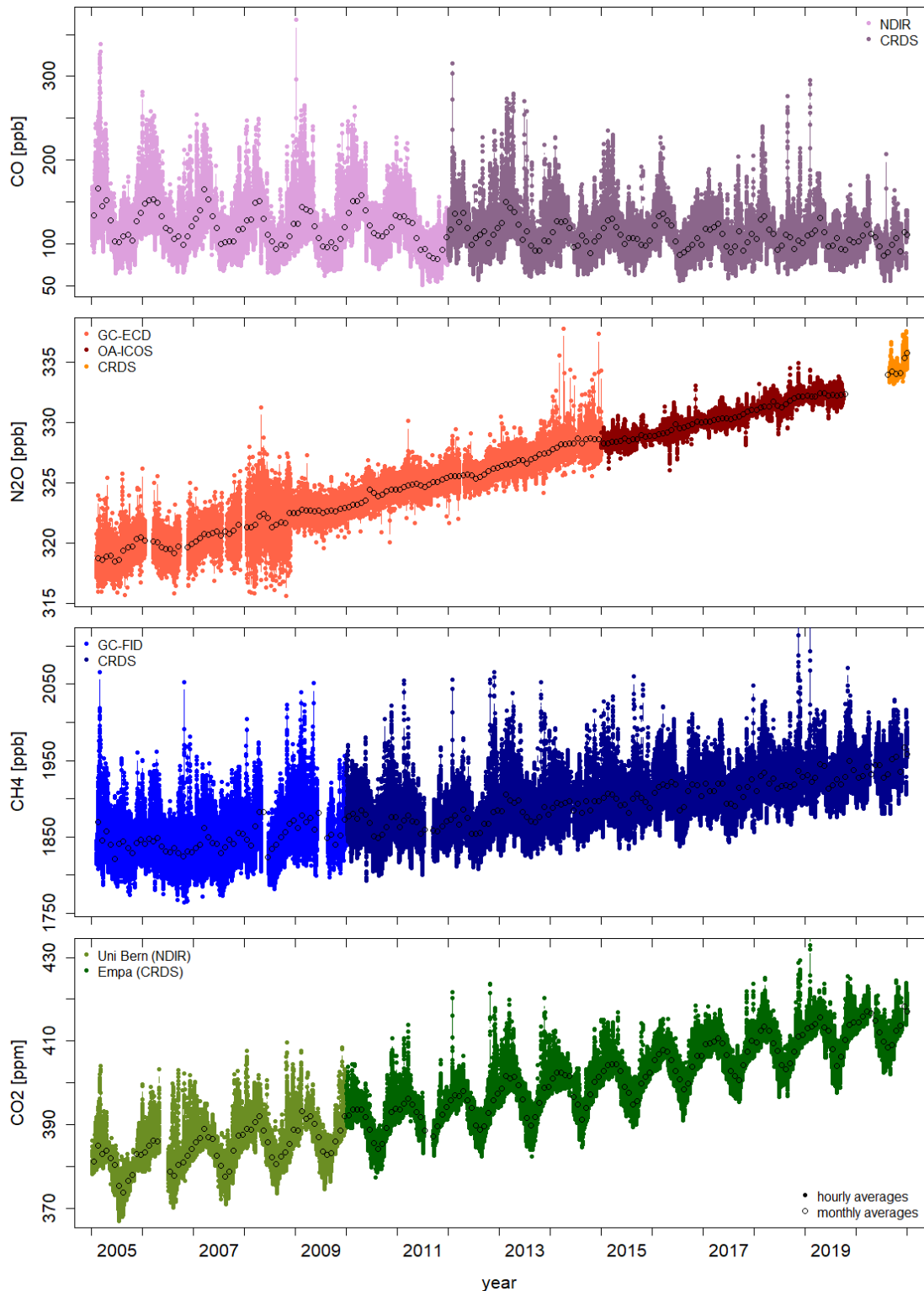
Abbildung 25: Zeitreihen der Stundenmittelwerte von CO 2 , CH 4 , N 2 O und CO auf dem Jungfraujoch. Offene Symbole stellen die Monatsmittel dar. Für CO 2 wurden die Messungen der Universität Bern im Januar 2010 durch Messungen der Empa ergänzt. Die CO 2 -Messungen der Universität Bern sind weiterhin operationell.
