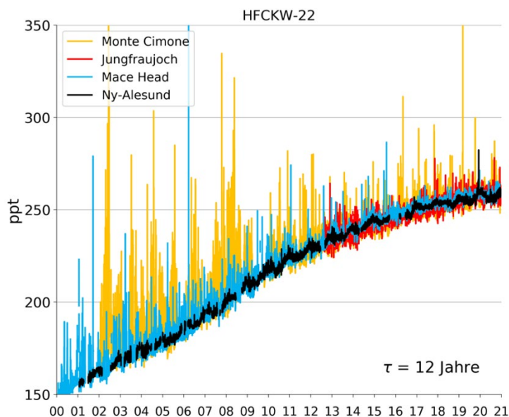
Abbildung 18: Zeitreihen von HFCKW-22 an vier europäischen Hintergrundstationen.
