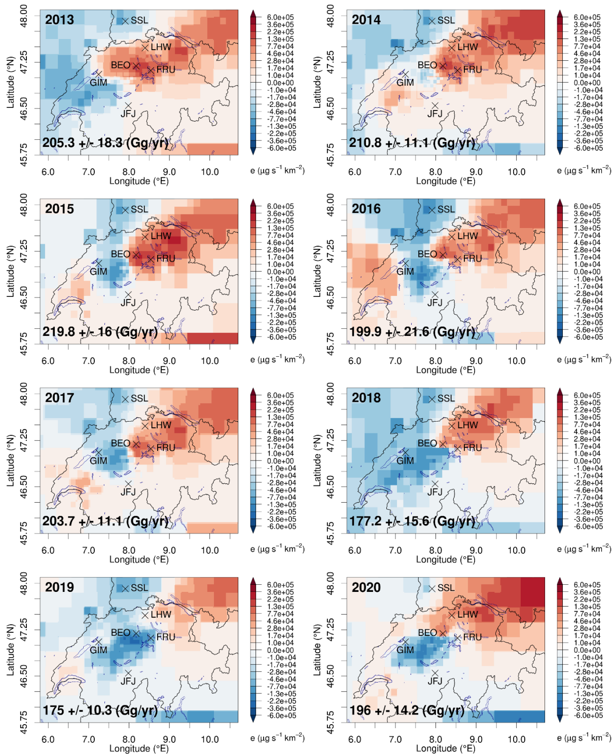
Abbildung 40: Räumliche Verteilung der Methanemissionsdifferenz der aus der inversen Modellierung gewonnenen Verteilung zur a-priori Verteilung des Inventars für die Jahre 2013 bis 2020. Dabei weisen blaue (rote) Regionen auf geringere (stärkere) Emissionen als im Inventar hin. Die Zahlen geben die totalen Schweizer Methanemissionen und deren Unsicherheit (1 \sigma -Level) des jeweiligen Jahres an.
