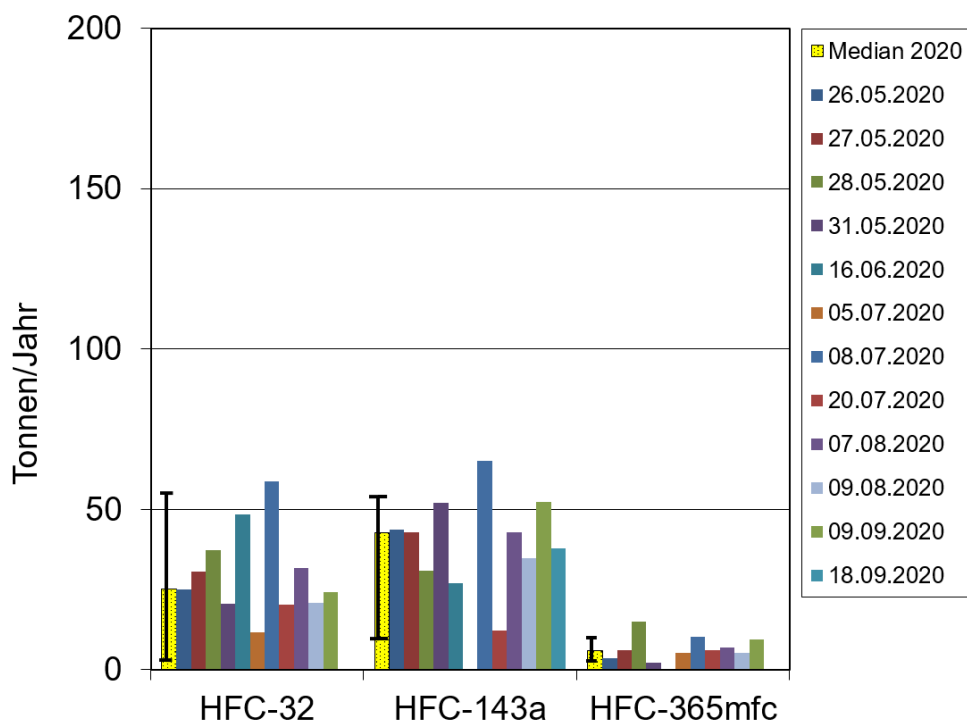
Abbildung A3: Grafische Darstellung der auf dem Jungfraujoch abgeschätzten Schweizer Emissionen der HFKW im Jahr 2020 an den 12 Tagen an welchen das Jungfraujoch vornehmlich unter Einfluss von Emissionen aus der Schweiz stand. Die jährliche Abschätzung entspricht dem Median.
