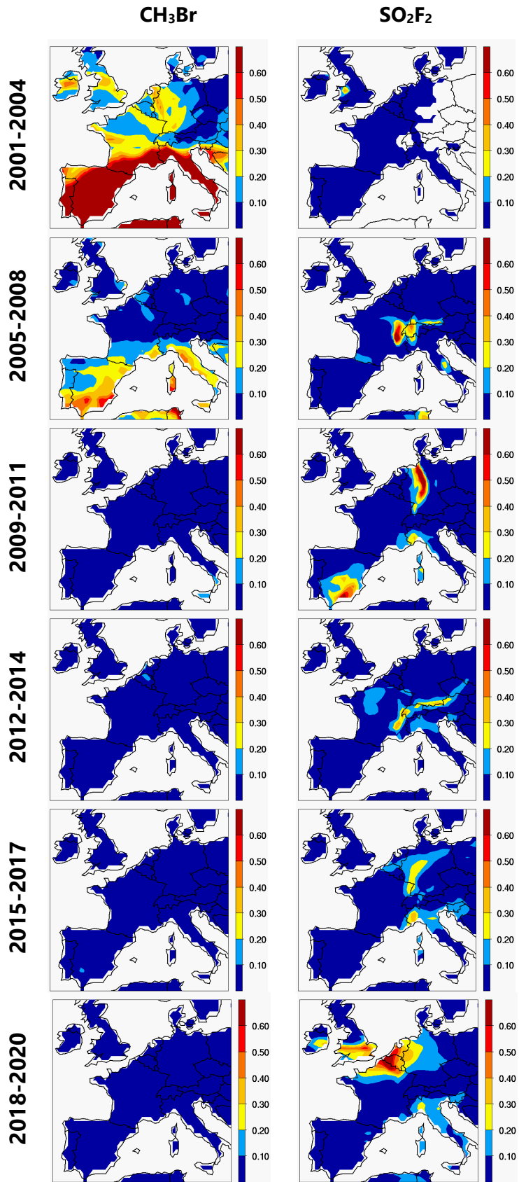
Abbildung 51: Analog zu Abbildung 47 für Methylbromid ( \text{CH}_3\text{Br} ) und \text{SO}_2\text{F}_2 .
