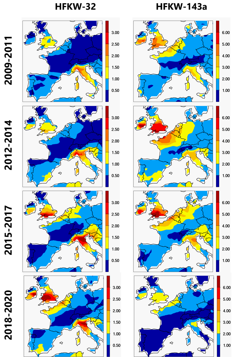
Abbildung 49: Analog zu Abbildung 47 für HFKW-32 und HFKW-143a, welche erst ab 2008 gemessen wurden.
