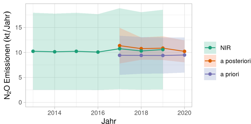
Abbildung 43: Zeitlicher Verlauf der Schweizer N_2O Emissionen: (grün, NIR) Treibhausgasinventar, (violett) als a priori verwendeter Startwert in der inversen Modellierung und (orange) Ergebnis (a posteriori) der inversen Modellierung. Die Unsicherheitsbänder geben das 2\sigma Konfidenzintervall der Jahresmittel an.
