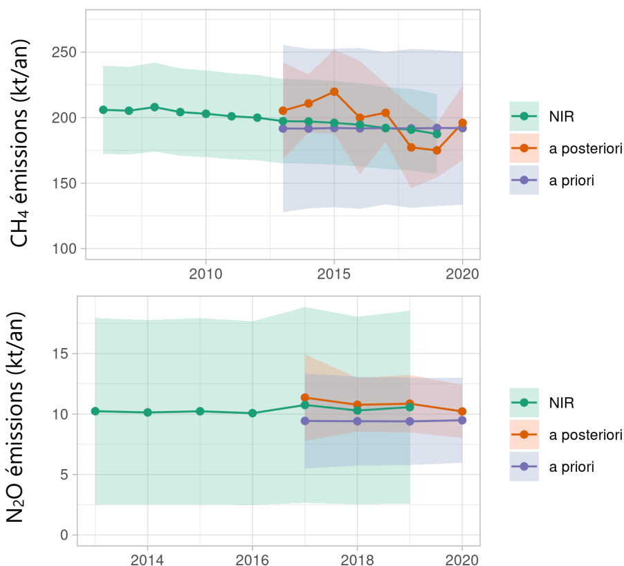
Figure S2: Evolution des émissions suisses de CH 4 (dessus) et N 2 O (dessous): Vert, inventaire suisse des gaz à effet de serre (NIR); violet, valeurs initiales (a priori) de la modélisation inverse; orange, résultats (a posteriori) de la modélisation inverse.
