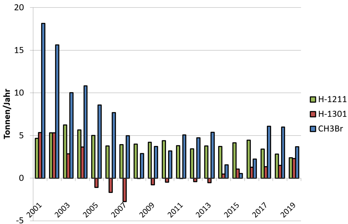
Abbildung 34: Mit Messungen auf dem Jungfrauoch abgeschätzte Schweizer Emissionen von ozonzerstörenden bromierten Substanzen, welche durch das Montrealer Protokoll reguliert sind (als arithmetisches Mittel über 3 Jahre).
