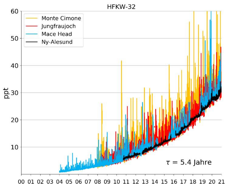
Abbildung 6: Zeitreihen von HFKW-32 an vier europäischen Hintergrundstationen.
