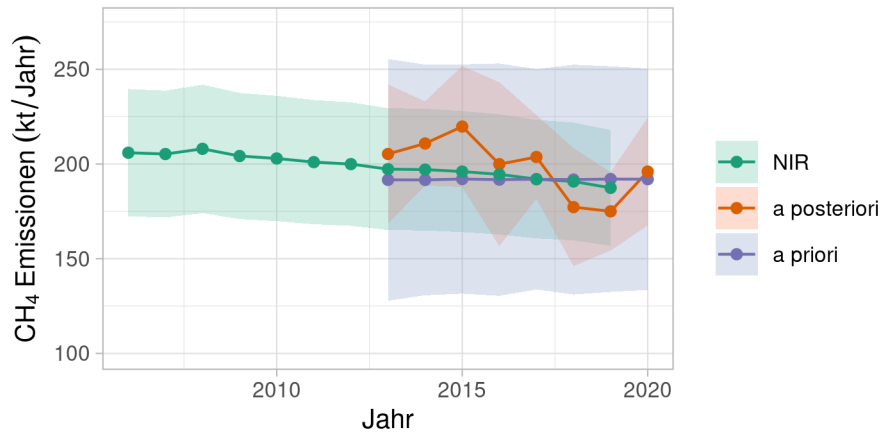
Abbildung 39: Zeitlicher Verlauf der Schweizer CH 4 Emissionen: (grün, NIR) Treibhausgasinventar, (violett) als a priori verwendeter Startwert in der inversen Modellierung und (orange) Ergebnis (a posteriori) der inversen Modellierung. Die Unsicherheitsbänder geben das 2 \sigma Konfidenzintervall der Jahresmittel an.
