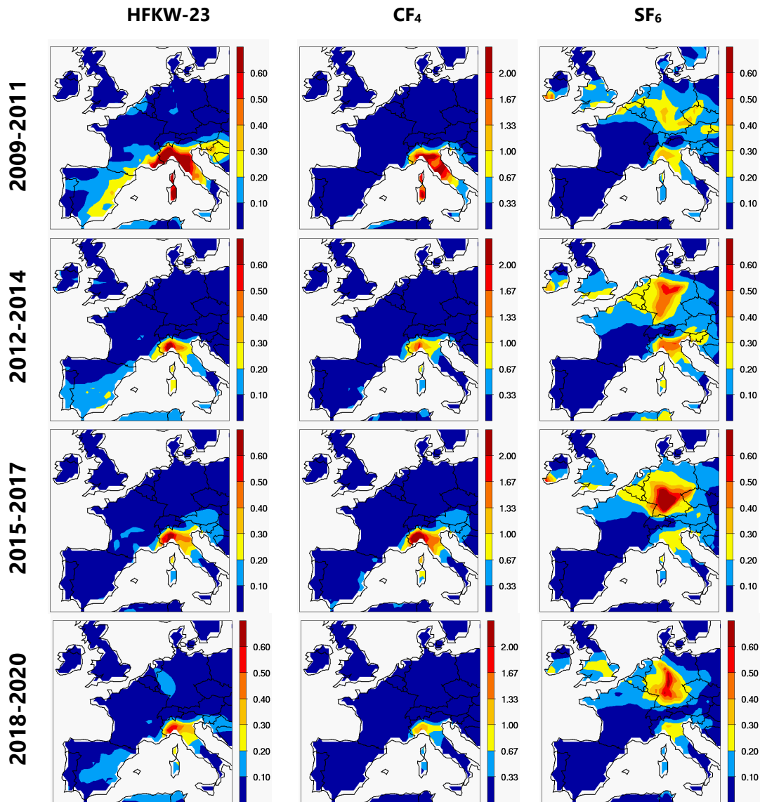
Abbildung 50: Analog zu Abbildung 47 für HFKW-23, CF 4 und SF 6 , welche erst ab 2008 genügend genau gemessen werden konnten.
