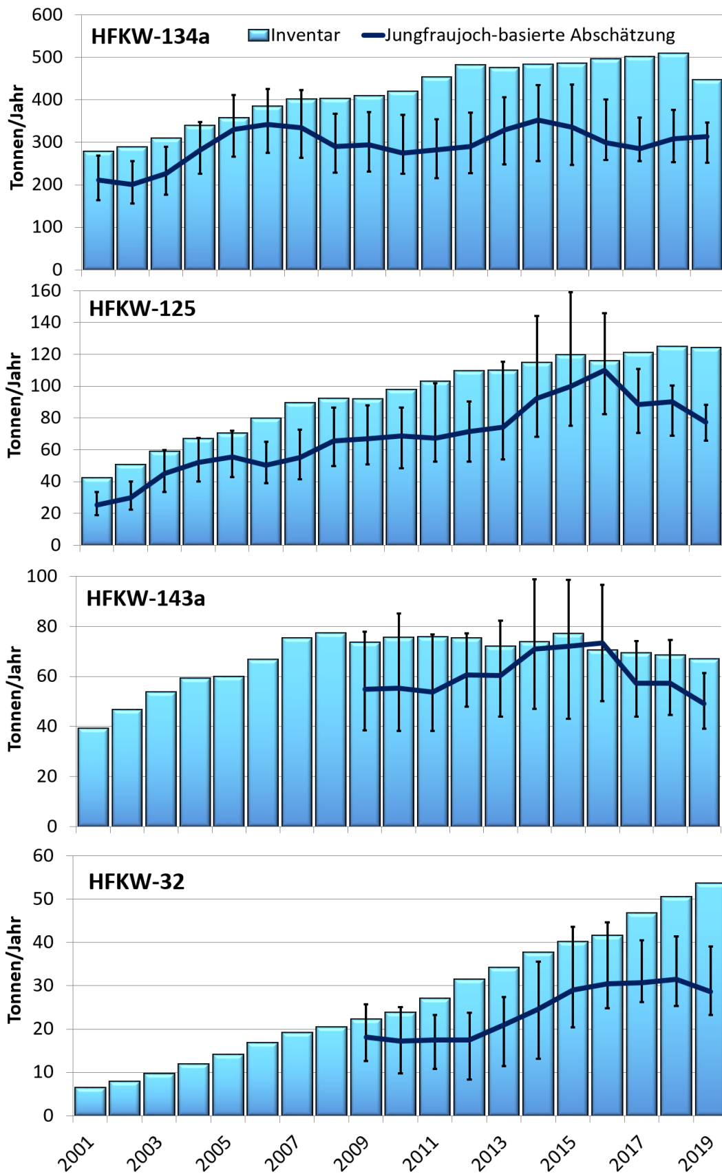
Abbildung 26: Vergleich der auf dem Jungfrauoch abgeschätzten Schweizer Emissionen von HFKW-134a, -125, -143a und -32 (inkl. 25%/75%-Quartile) mit den Werten aus dem Inventar. Diese Substanzen werden vorwiegend in Kälteanlagen eingesetzt.
