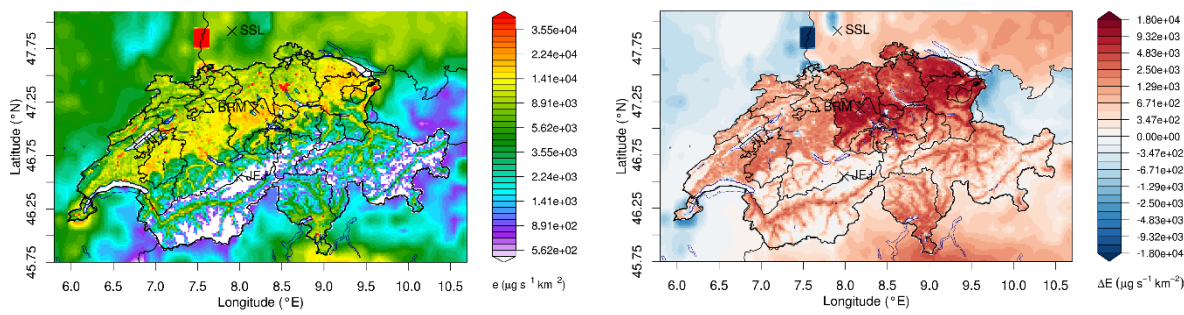
Abbildung 44: (links) Räumliche Verteilung der Schweizer N_2O Emissionen nach MeteoTest Inventar und (rechts) Emissionsdifferenz der aus der inversen Modellierung gewonnenen Verteilung als Mittel für die Jahre 2017-2020. Dabei weisen blaue (rote) Regionen auf geringere (stärkere) Emissionen als im Inventar hin.
