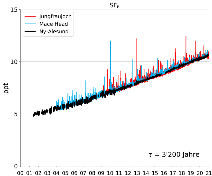
Abbildung 14: Zeitreihen von SF 6 an drei europäischen Hintergrundstationen.
