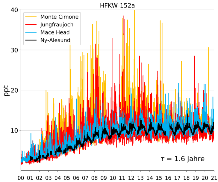
Abbildung 7: Zeitreihen von HFKW-152a an vier europäischen Hintergrundstationen
