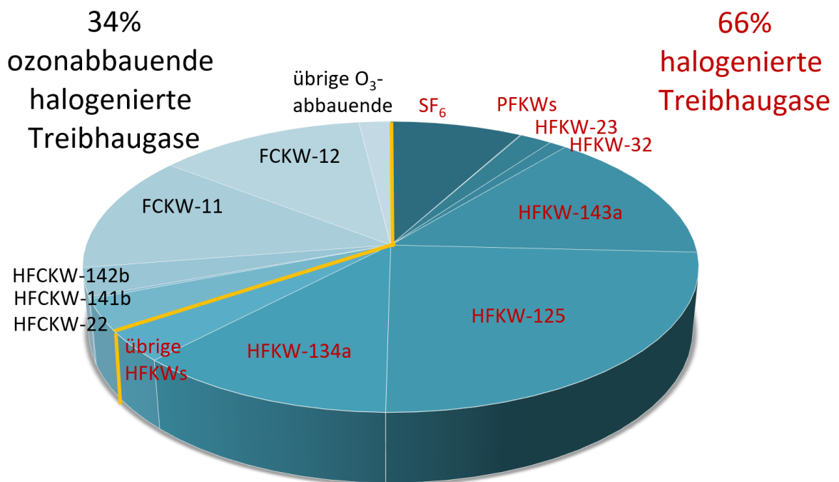
Abbildung 36: Summe der klimarelevanten Schweizer Emissionen in 2019 (als CO 2 -Äquivalente) von halogenierten Verbindungen, welche nur Treibhausgase sind (HFKWs, PFKWs, SF 6 ) im Vergleich mit der Summe der halogenierte Verbindungen welche zusätzlich noch eine ozonabbauende Wirkung haben (FCKWs, HFCKWs, Halone, Methylbromid, chlorierte Lösungsmittel).
