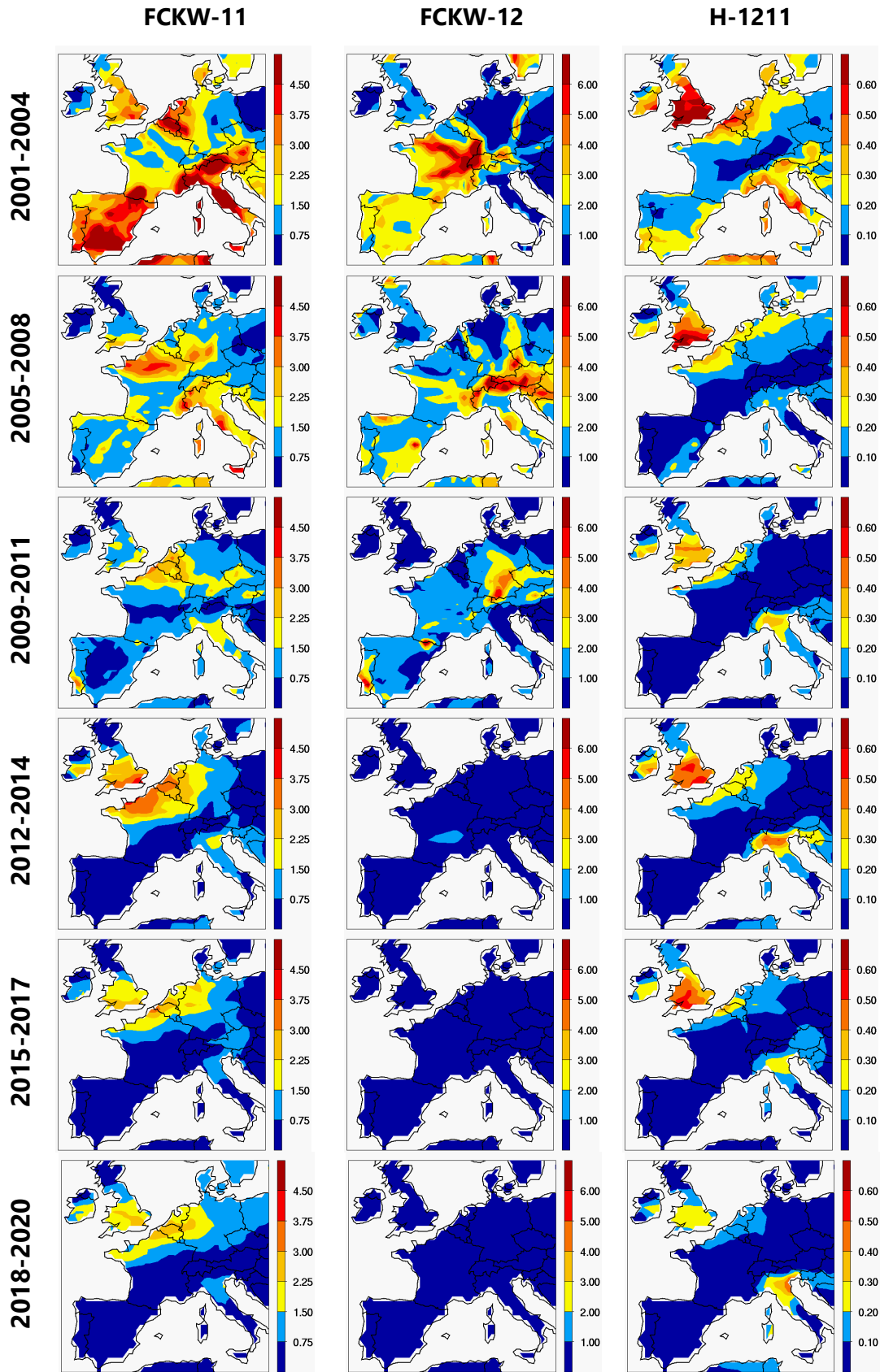
Abbildung 52: Analog zu Abbildung 47 für FCKW-11, FCKW-12 und Halon-1211.
