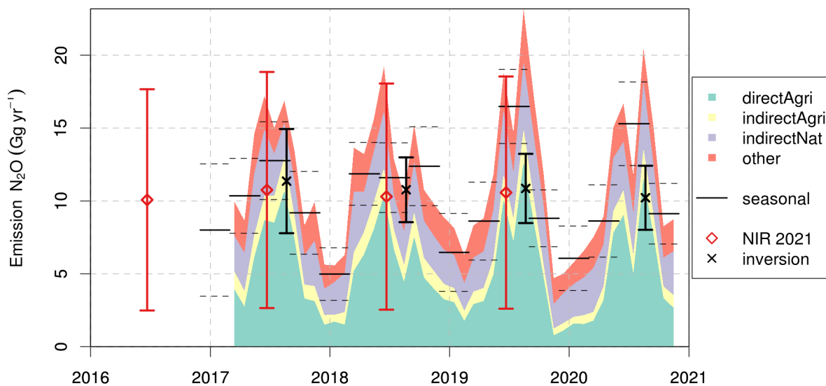
Abbildung 46: Zeitlicher Verlauf der aus der Inversion bestimmten monatlichen Schweizer Lachgas Emissionen (schattierte Flächen; grün: Landwirtschaft direkt, gelb: Landwirtschaft indirekt, violett: (semi-)natürliche Flächen indirekt, orange: andere) als Mittel über alle Sensitivätsinversionen mit monatlicher Auslösung. Horizontale Linien geben die a posteriori Emissionen aller saisonalen Inversionen (Mittel: durchgezogene Linien, Unsicherheit: gestrichelte Linien). Jahresmittel des Inventars und über alle a posteriori Emissionen sind als Symbole mit Fehlerbalken gegeben (horizontal versetzt für bessere Sichtbarkeit). Alle Unsicherheiten sind auf dem 2- \sigma Niveau angegeben.
