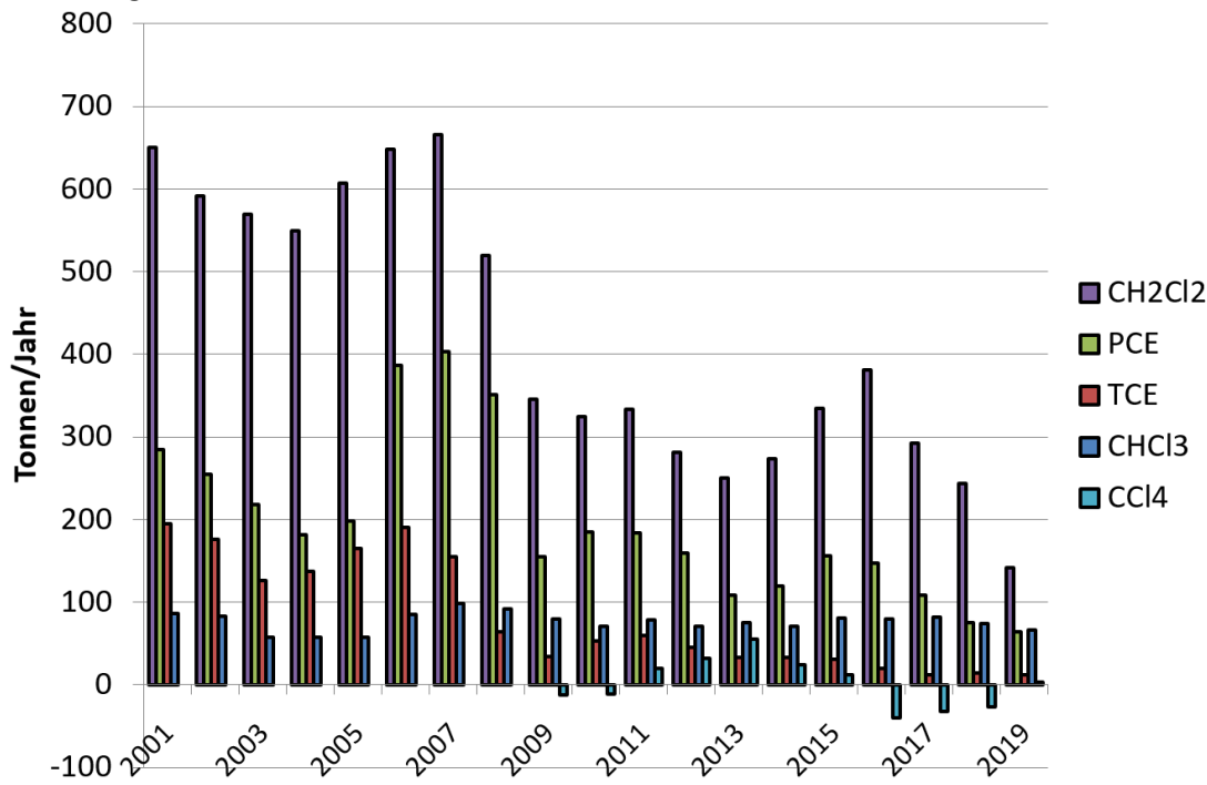
Abbildung 35: Mit Messungen auf dem Jungfraujoch abgeschätzte Schweizer Emissionen von chlorierten Lösungsmitteln (als arithmetisches Mittel über 3 Jahre).
