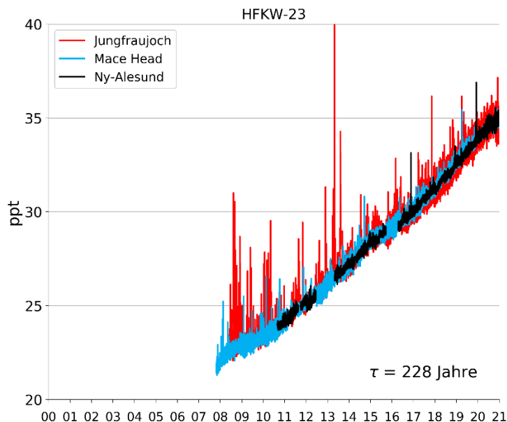
Abbildung 11: Zeitreihen von HFKW-23 an drei europäischen Hintergrundstationen.
