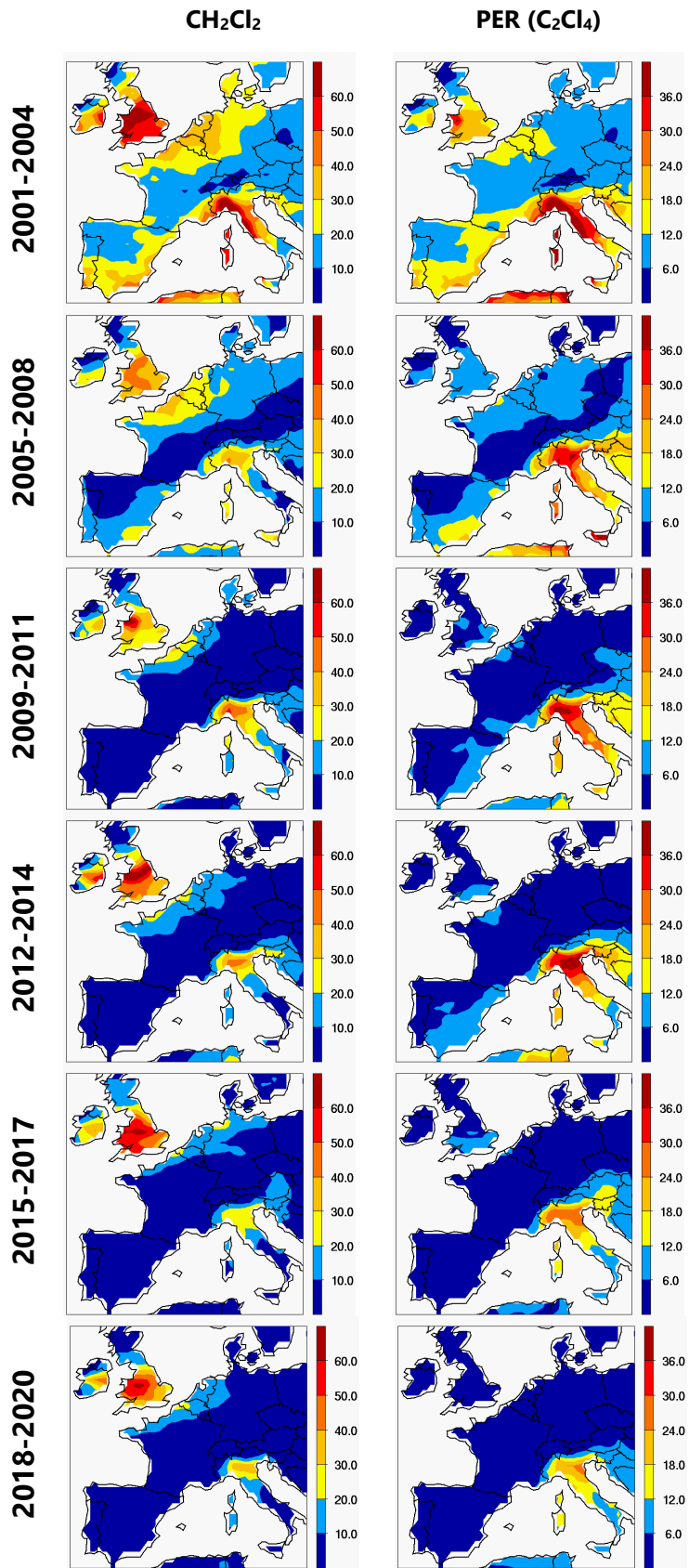
Abbildung 53: Analog zu Abbildung 47 für die chlorierten Lösemittel Dichlormethan ( \text{CH}_2\text{Cl}_2 ) und Perchloroethylen ( \text{C}_2\text{Cl}_4 )
