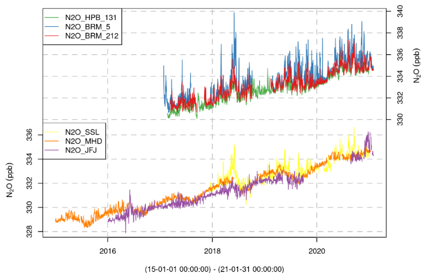
Abbildung 42: Zeitserie der täglichen Mittelwerte der N 2 O Konzentrationen an den in der inversen Modellierung verwendeten Stationen Beromünster (BRM: Messhöhen 5 m und 212 m über Grund, blau, rot), Jungfrauoch (violett) und Schauinsland (gelb) und den zusätzliche Hintergrundstationen Mace-Head (orange) und Hohenpeissenberg (grün).
