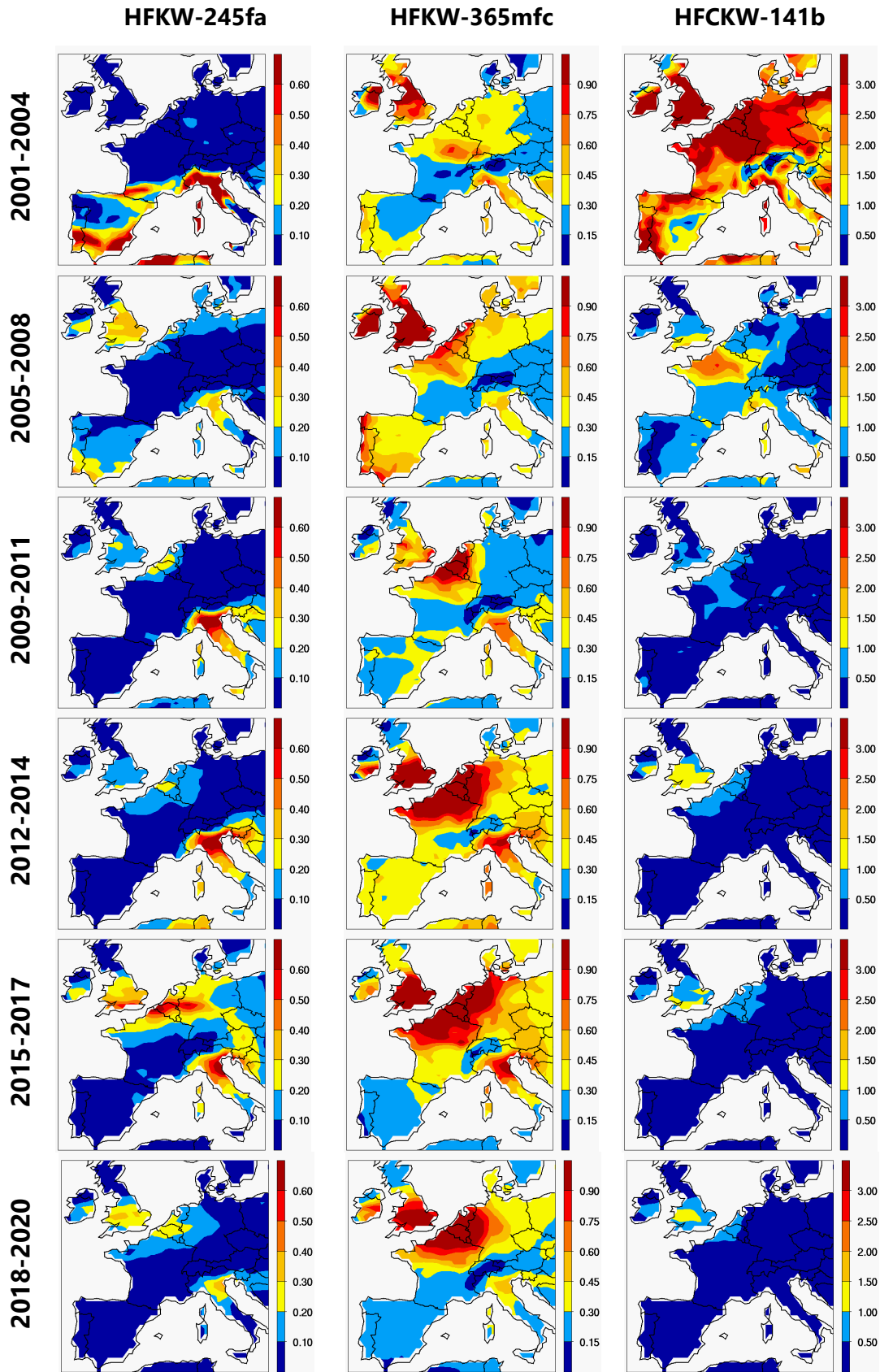
Abbildung 48: Analog zu Abbildung 47 für HFKW-245fa, HFKW-365mfc und HFCKW-141b.
