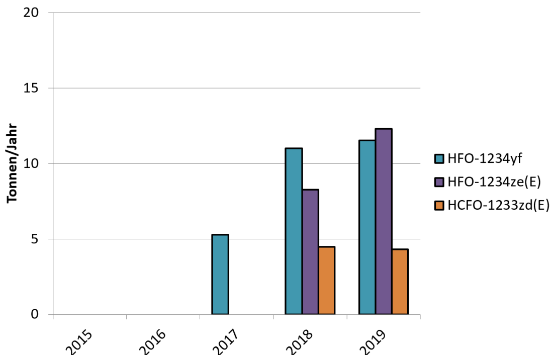
Abbildung 31: Jungfraujoch-basierte Emissionsabschätzung der HFO-1234yf, HFO-1234ze(E) und HCFO-1233zd(E).
