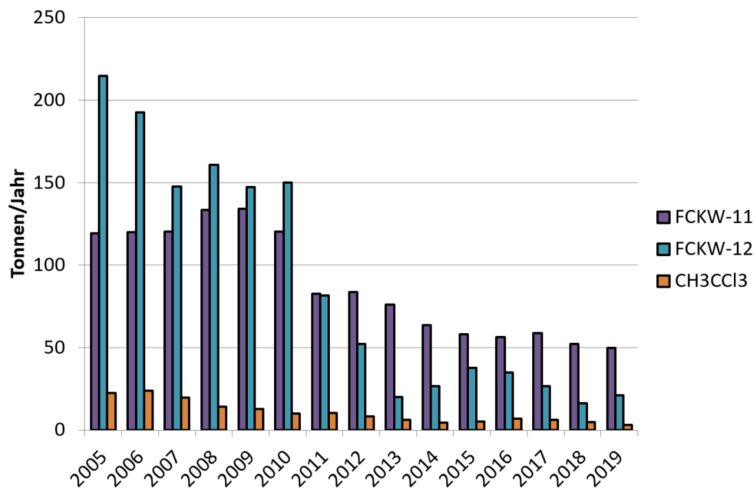
Abbildung 32: Jungfraujoch-basierte Emissionsabschätzung der FCKW-11 und -12 sowie von 1,1,1-Trichlorethan (CH 3 CCl 3 ).
