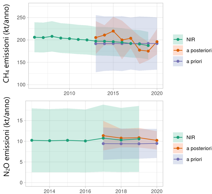
Immagine S2: Evoluzione delle emissioni di CH 4 (sopra) e di N 2 O (sotto) in Svizzera: Verde, NIR; National Inventory Report) inventario dei gas serra; viola, come valore a priori utilizzato nella modellazione inversa; arancione, risultato (a posteriori) della modellazione inversa.
