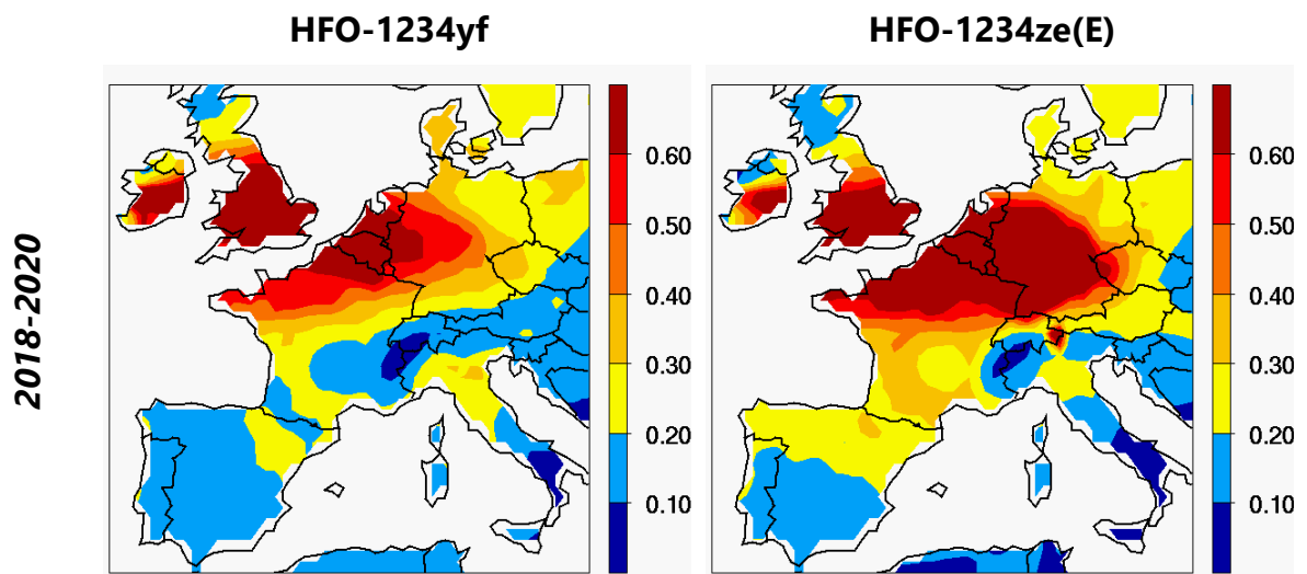
Abbildung 54: Analog zu Abbildung 47 für HFO-1234yf und HFO-1234ze(E).
