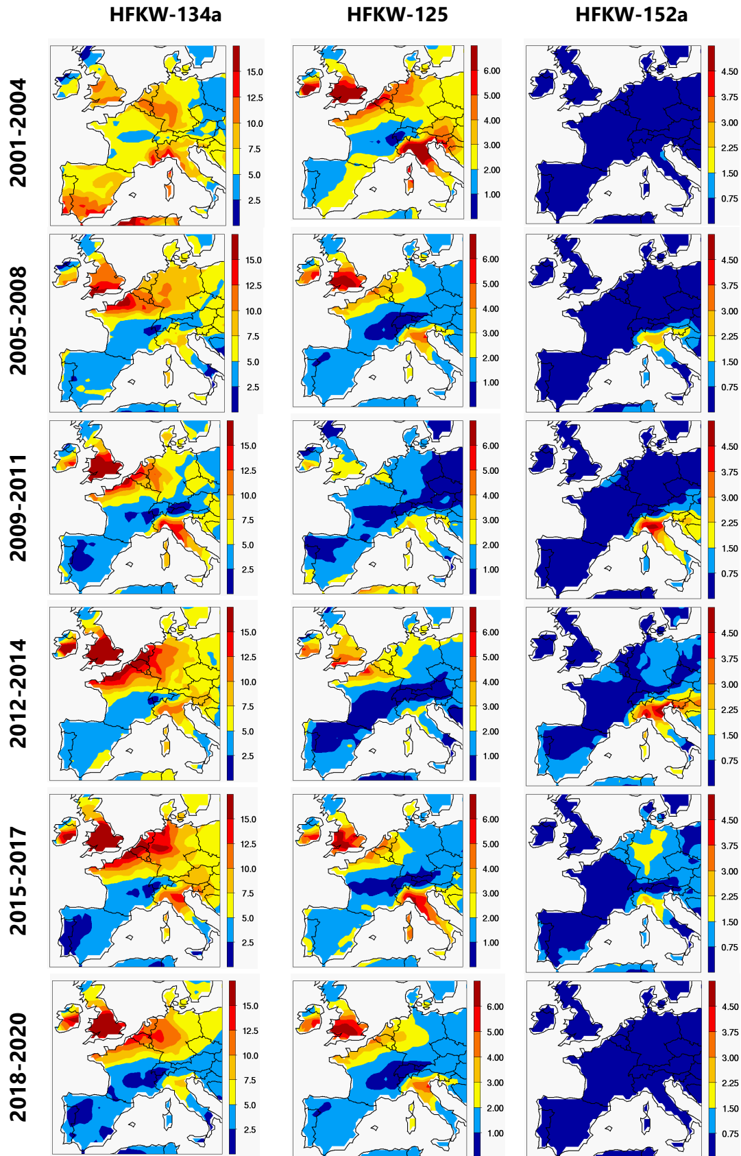
Abbildung 47: Potentielle europäische Quellregionen von HFKW-134a, -125, -152a. Die Werte bezeichnen Emissionsraten in Einheiten von \text{kg km}^{-2} \text{Jahr}^{-1} .
