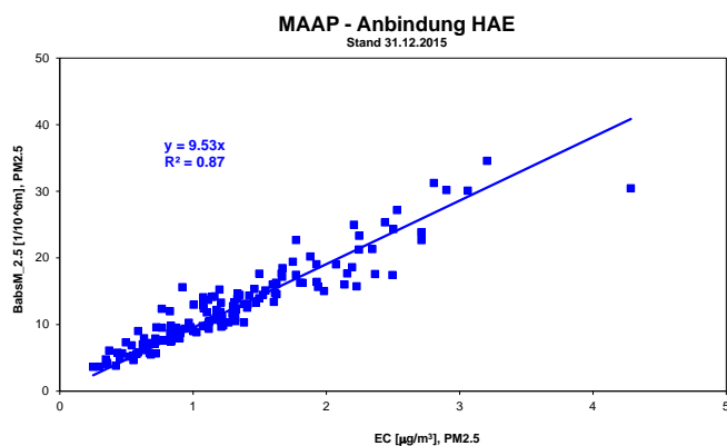
Abb. A4-2: Vergleich von kontinuierlichen MAAP-Messungen mit EC-Messungen (TOT Messungen) am Standort Härkingen (Messperiode: 1.1.2011 - 31.12.2015)
