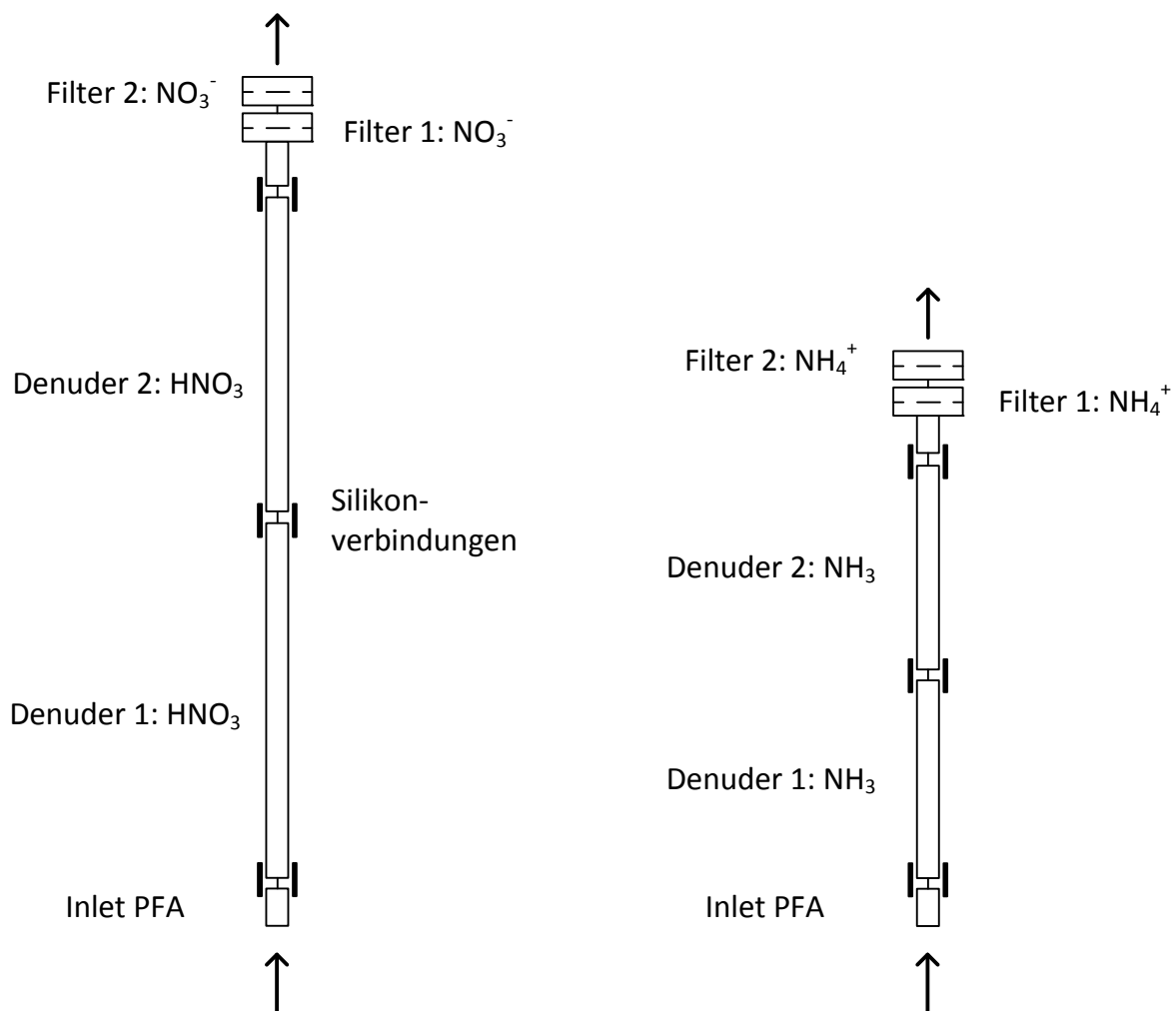
Abb. 3-32: Probetrains zur getrennten Bestimmung von \text{HNO}_3 , \text{NO}_3^- und \text{NH}_3 , \text{NH}_4^+
