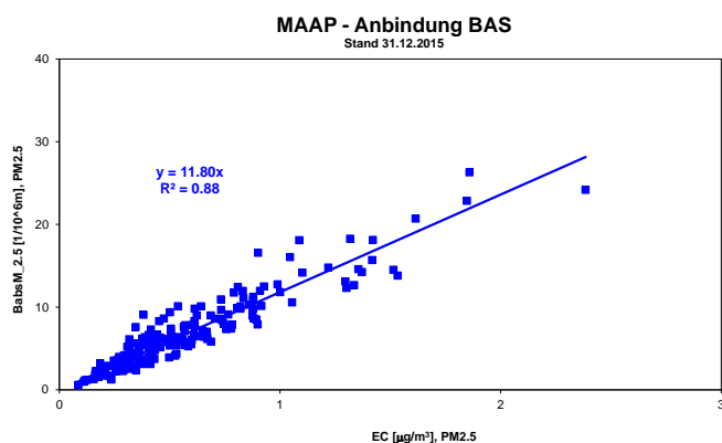
Abb. A4-1: Vergleich von kontinuierlichen MAAP-Messungen mit EC-Messungen (TOT Messungen) am Standort Basel (Messperiode: 16.2.2008 - 31.12.2015)
