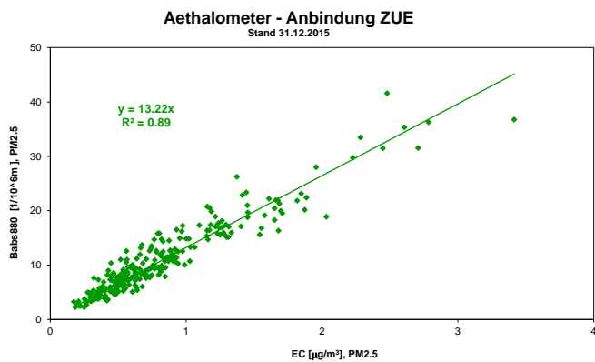
Abb. A4-7: Vergleich von kontinuierlichen Aethalometer-Messungen mit EC-Messungen (TOT Messungen) am Standort Zürich (Messperiode: 3.4.2009 - 31.12.2015)
