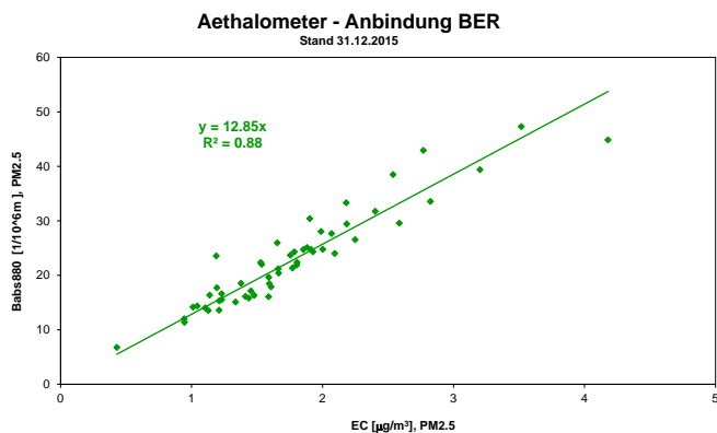
Abb. A4-8: Vergleich von kontinuierlichen Aethalometer-Messungen mit EC-Messungen (TOT Messungen) am Standort Bern (Messperiode: 12.12.13 - 31.12.2015)
