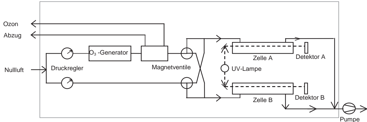
Abb. 4-5: Schematische Darstellung des Thermo 49C-PS
