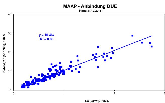
Abb. A4-4: Vergleich von kontinuierlichen MAAP-Messungen mit EC-Messungen (TOT Messungen) am Standort Dübendorf (Messperiode: 1.1.2011 - 31.12.2015)
