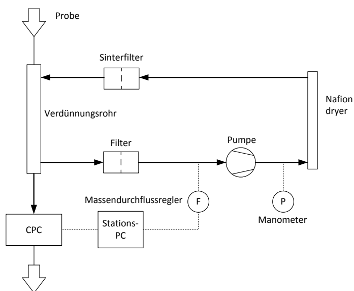
Abb. 3-25: CPC-Verdünnungseinheit
