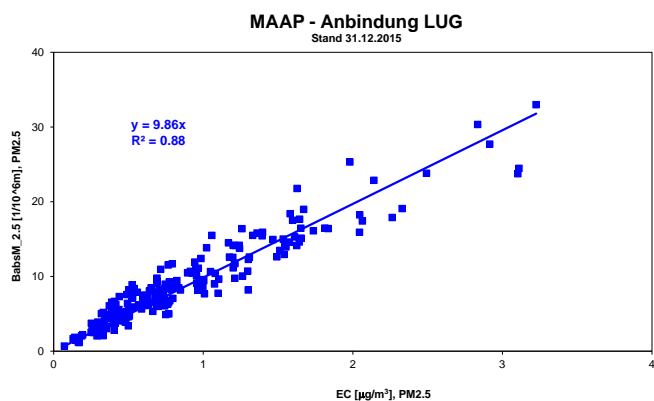
Abb. A4-3: Vergleich von kontinuierlichen MAAP-Messungen mit EC-Messungen (TOT Messungen) am Standort Lugano (Messperiode: 1.1.2011 - 31.12.2015)
