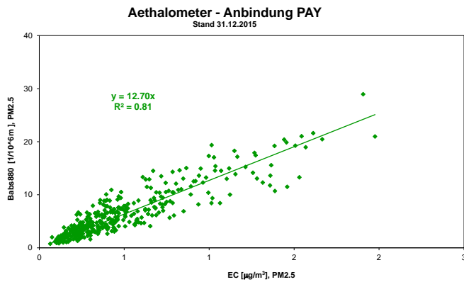
Abb. A4-6: Vergleich von kontinuierlichen Aethalometer-Messungen mit EC-Messungen (TOT Messungen) am Standort Payerne (Messperiode: 23.3.2008 - 31.12.2015)
