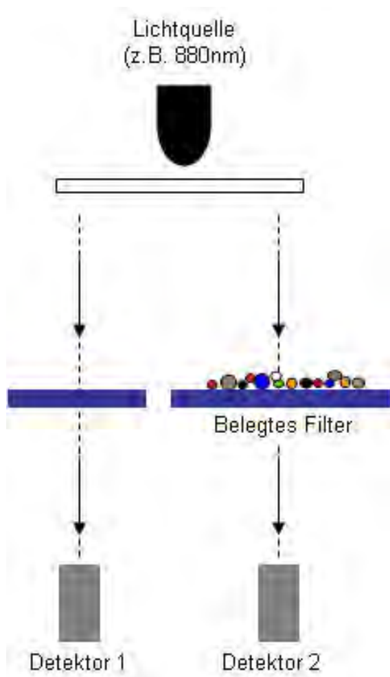
Abb. 3-24: Schematischer Geräteaufbau eines Russmonitor Magee Aethalometer AE31
