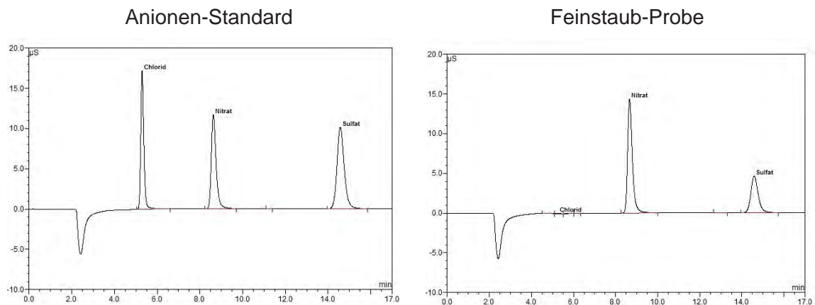
Abb. 3-22: IC-Chromatogramm von Anionen-Standard und Feinstaub-Probe
