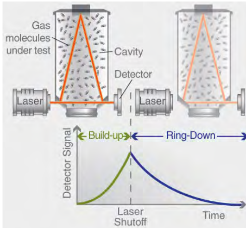
Abb. 3-12: Schematische Darstellung des Cavity Ring Down Spektrometers (Quelle: www.picarro.com )
