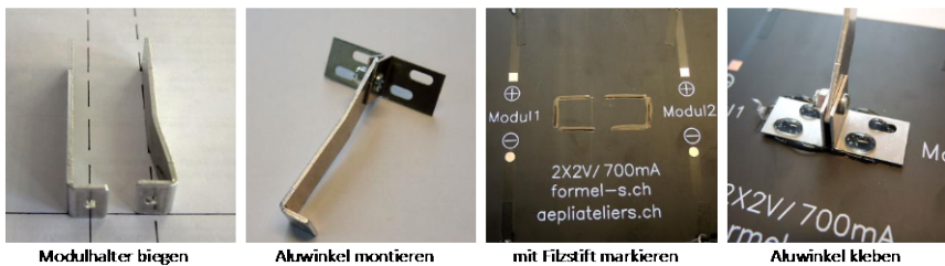
Modulhalter biegen
